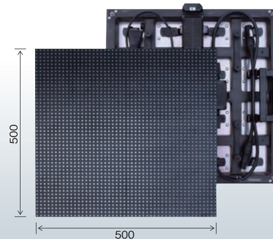
■ i-max Floor 5w-m2 LEDスクリーン (単位:mm)
