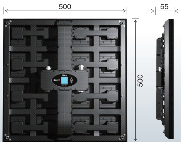
■ i-max Floor 10w LEDスクリーン (単位:mm) 1パネルあたりの寸法図
