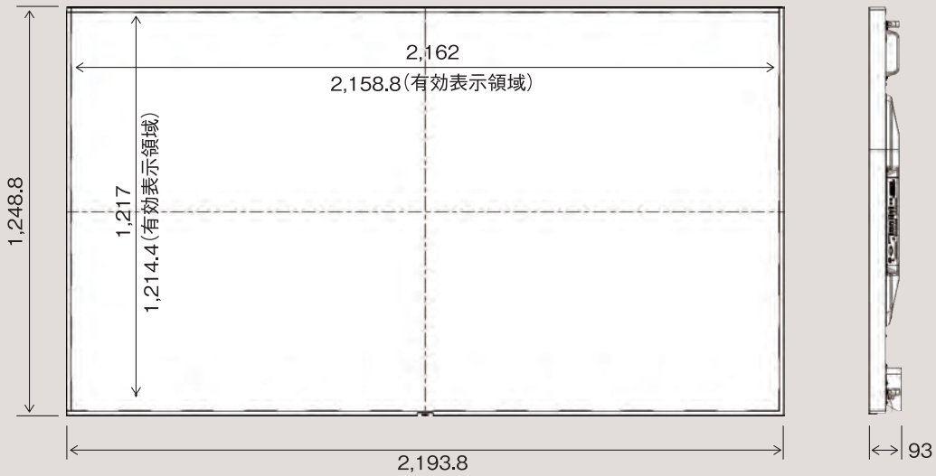
98型マルチシンク液晶ディスプレイ (外形図)
