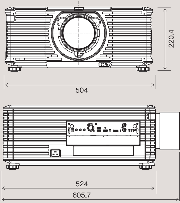
BARCO I600-4K15 サイズ表 (本体)
