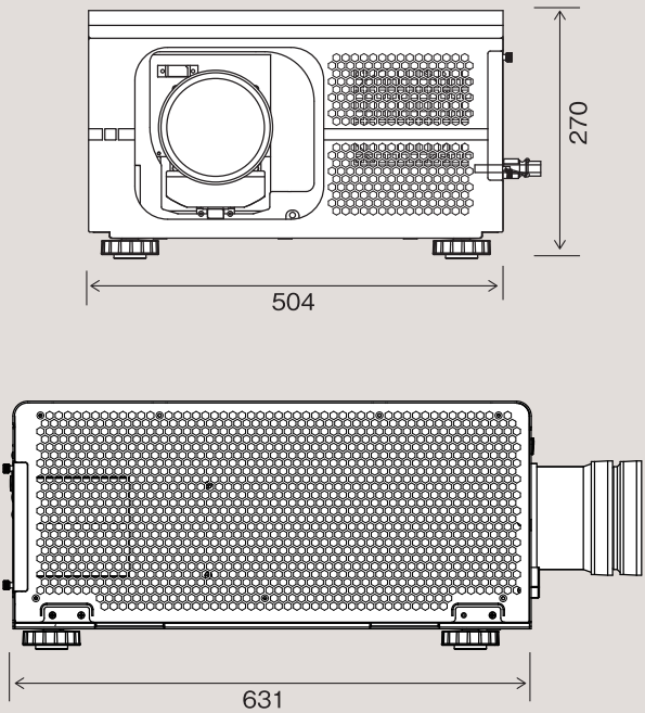
BARCO RLM-W14 サイズ表 (本体)
