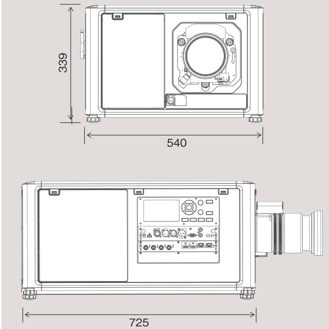
BARCO UDM-4K22 サイズ表(本体) (単位:mm)
