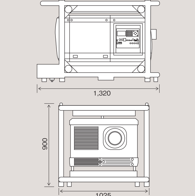
BARCO HDQ-2K40 サイズ表(本体) (単位:mm)
