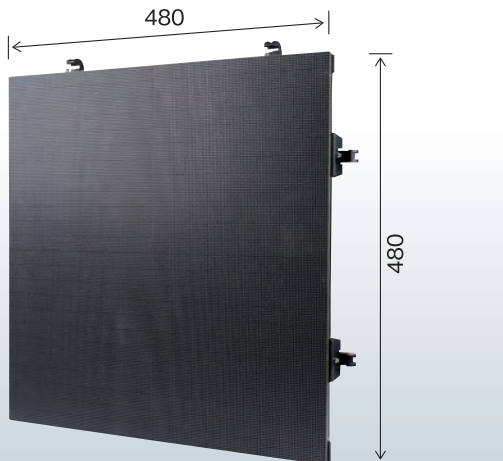
■ ACTIV 2.8 LEDスクリーン 1パネルあたりの寸法図
