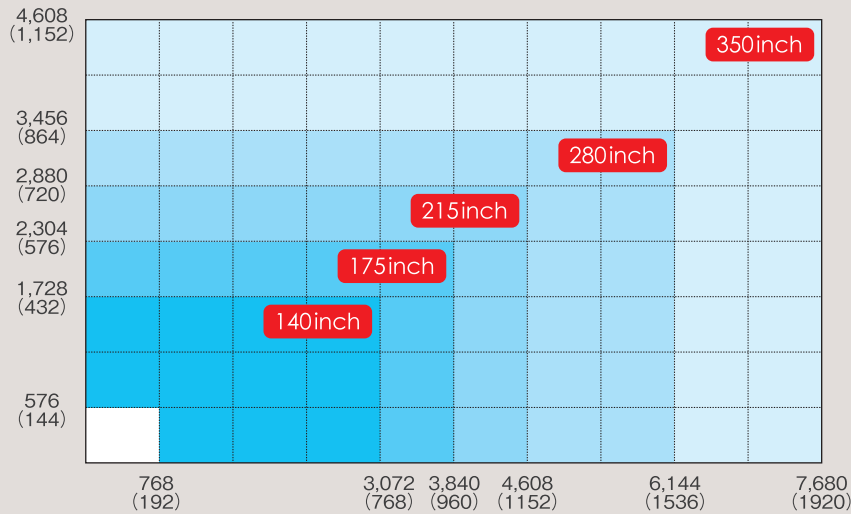
■ アクティブ 4 LEDスクリーン / 1パネルあたりの仕様
