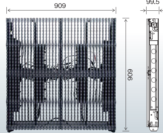
■ i-max 25w LEDスクリーン 1パネルあたりの寸法図
