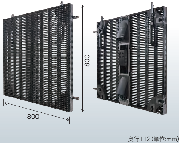
■ i-max 9 LEDスクリーン 1パネルあたりの寸法図
