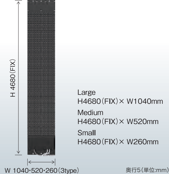
■ i-max Ultra Light 10w LEDスクリーン (単位:mm) 1パネルあたりの寸法図
