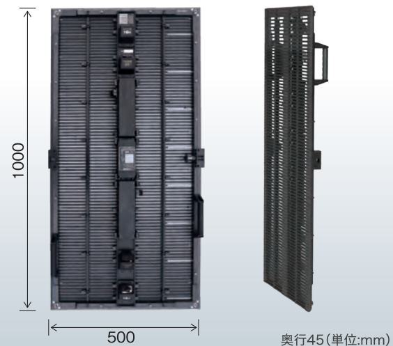
■ i-max Light 10w-m3 LEDスクリーン (単位:mm) 1パネルあたりの寸法図
