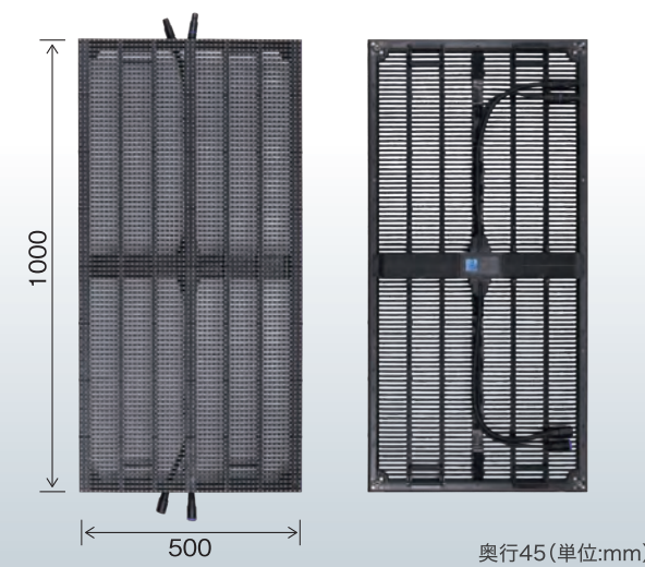
■ i-max Light 10w LEDスクリーン (単位:mm) 1パネルあたりの寸法図
