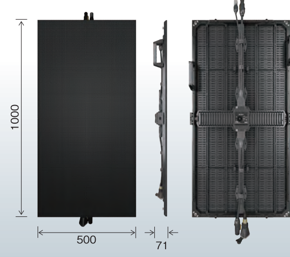
■ i-max Light 5w-m3 DRC LEDスクリーン (単位:mm) 1パネルあたりの寸法図
