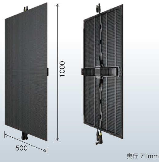
■ i-max Light 5w-m2 LEDスクリーン (単位:mm) 1パネルあたりの寸法図
