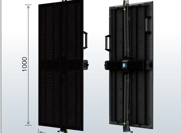
■ i-max Light 5w-m1 LEDスクリーン (単位:mm) 1パネルあたりの寸法図
