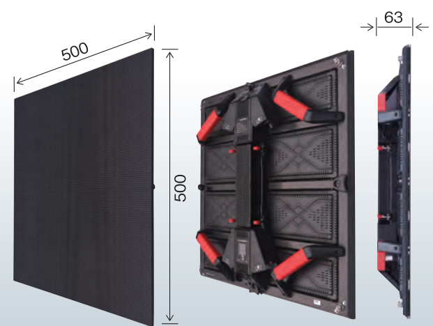
■ i-max Light 3w-m2 LEDスクリーン (単位:mm) 1パネルあたりの寸法図
