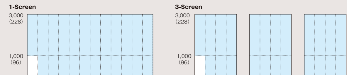
《i-max Light 10w / i-max Light 10w-m3 サイズ構成(有効サイズ)活用例》 (単位:mm / ( )内 pixel)
