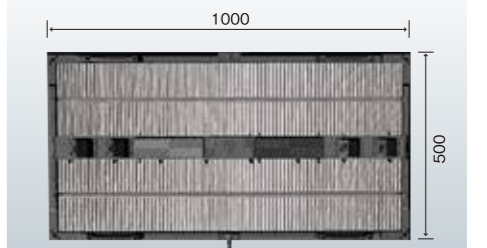
■ i-max Light 10w-m3 LEDスクリーン (単位:mm) / 1パネルあたりの寸法図
