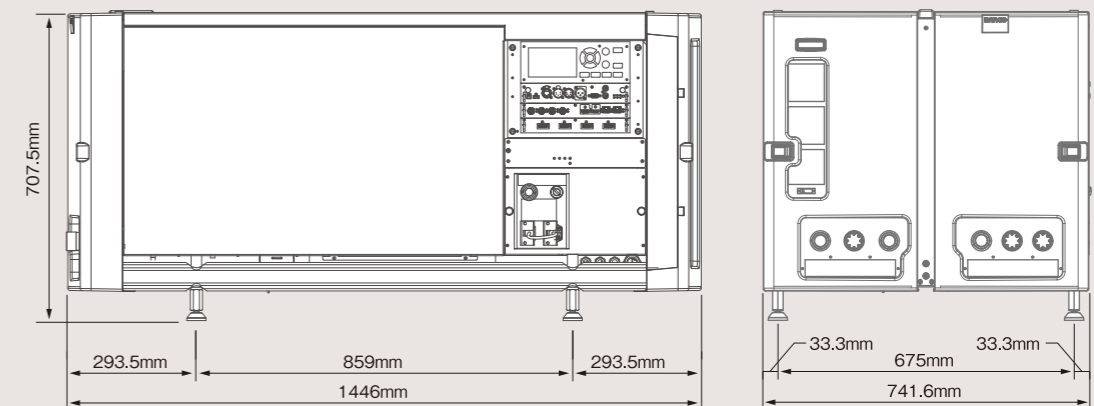
■ BARCO XDL-4K75 サイズ表(本体)
