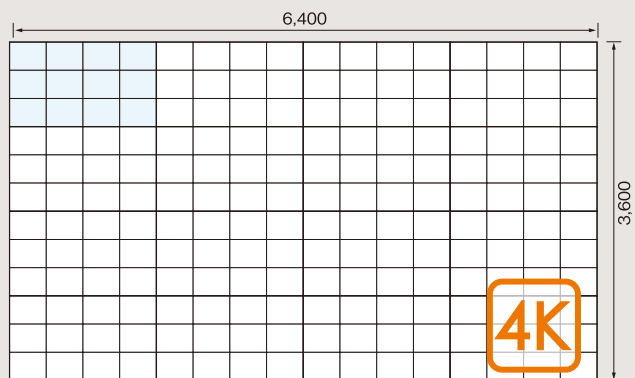
■ ACTIV-1.6 4K・289インチパネル寸法図
